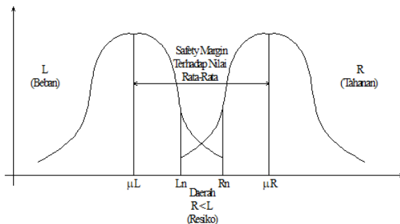
Gambar 6. Penentuan Daerah Risiko Akibat Beban Dan Tahanan
