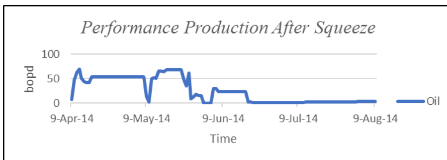
Gambar 15 Performance Produksi Setelah Squeeze Cementing dan Penambahan Perforasi
